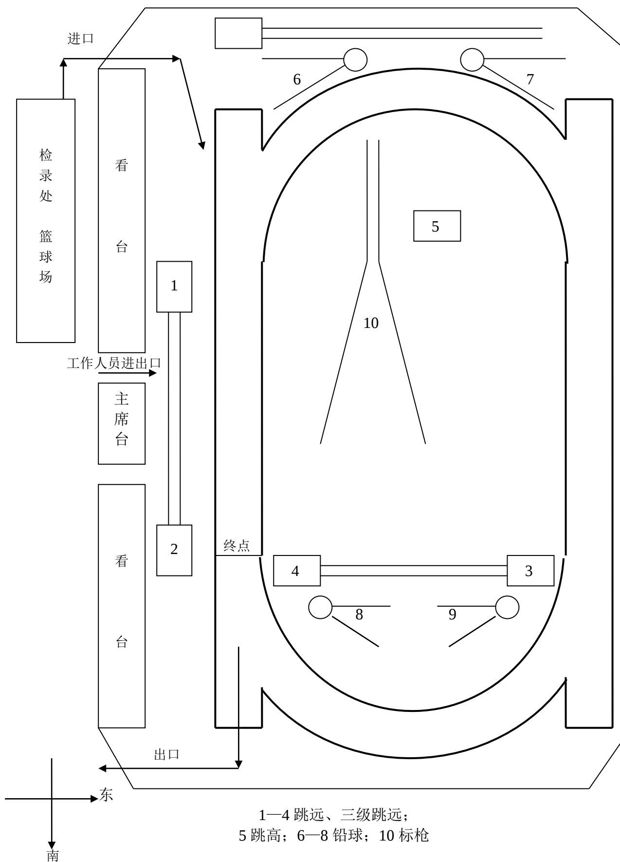
田径运动场地平面图
